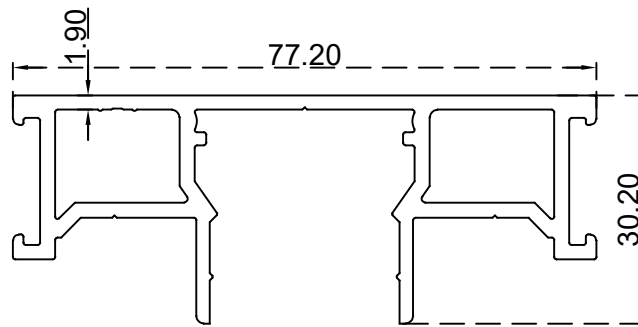
حلق تقطيع مكاتب 77.2*30.2 ملم الرقم التسلسلي للصنف: AS00099 الوزن 1.226:(Kg/m)
