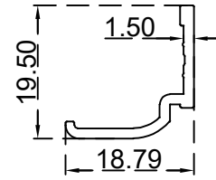
كليس دفة الرقم التسلسلي للصنف: AS00059 الوزن 1.130:(Kg/m)
