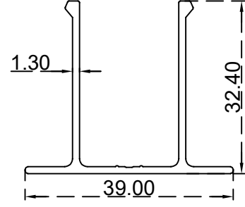
تحويله حلق لزجاج دبل الرقم التسلسلي للصنف: AS00068 الوزن 0.378:(Kg/m)
