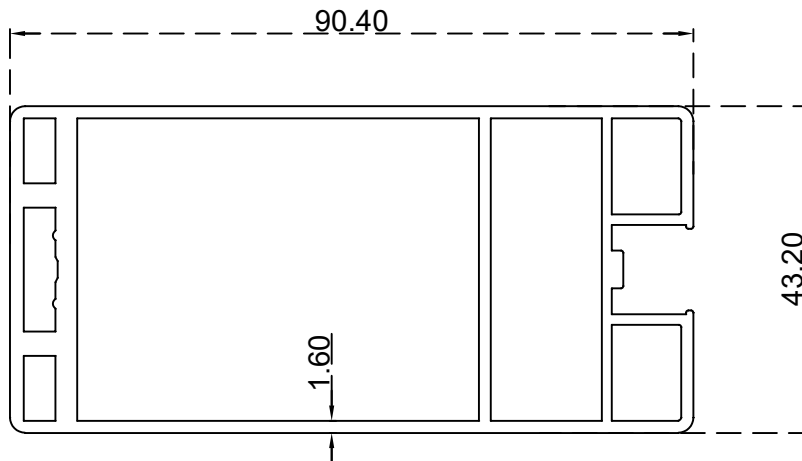
دفة باب رئيسي الرقم التسلسلي للصنف: AS00056 الوزن 1.872:(Kg/m)
