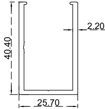
يو زجاج 40.4*25.7 ملم الرقم التسلسلي للصنف: AS00070 الوزن 0.600:(Kg/m)
