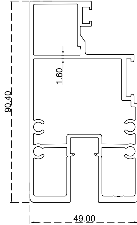
تحتون دفة باب الرقم التسلسلي للصنف: AS00098 الوزن 2.007:(Kg/m)
