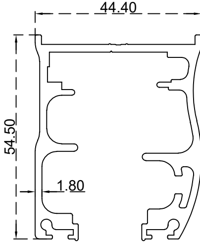
عليون تحتون تلسكوب الرقم التسلسلي للصنف: AS00062 الوزن 1.418:(Kg/m)
