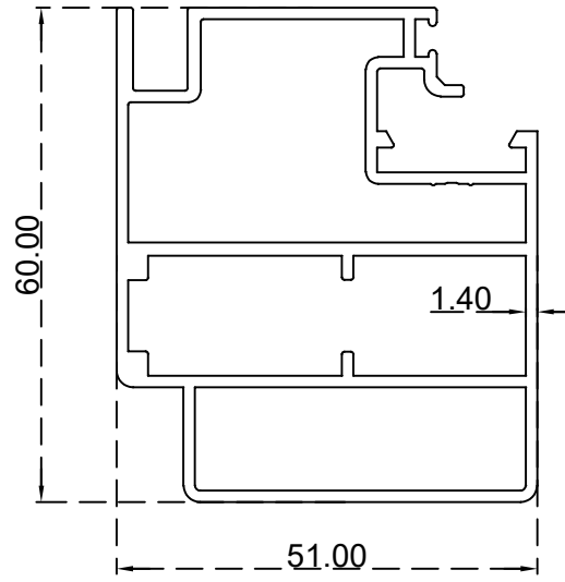
دفة باب عازلة للصوت الرقم التسلسلي للصنف: AS00057 الوزن 1.419:(Kg/m)
