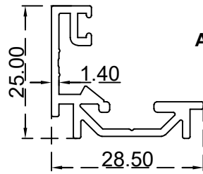
يو ارضية 28.5 ملم الرقم التسلسلي للصنف: AS00054 الوزن 0.368:(Kg/m)
