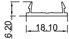
غطاء حلق الرقم التسلسلي للصنف: AS00042 الوزن 0.090: (Kg/m)
