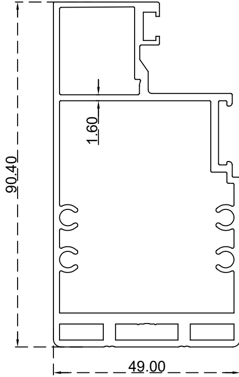
جانب عليون دفة باب الرقم التسلسلي للصنف: AS00097A الوزن 2.012:(Kg/m)
