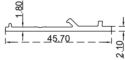
كلبس حلق دفعة تقطيع مكاتب الرقم التسلسلي للصنف: AS00072 الوزن 0.277:(Kg/m)
