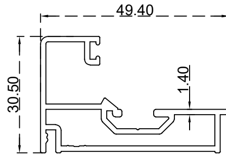
يو ارضية 47 ملم الرقم التسلسلي للصنف: AS00053 الوزن 0.699:(Kg/m)
