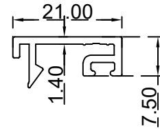
كليس زجاج 7.5 ملم الرقم التسلسلي للصنف: AS00051 الوزن 0.183:(Kg/m)
