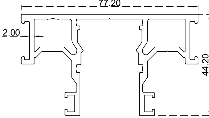
حلق تقطيع مكاتب 44.2*77.2 ملم الرقم التسلسلي للصنف: AS00067 الوزن 1.552:(Kg/m)
