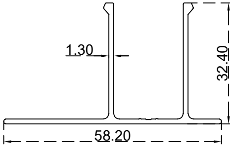
تحويله حلق لزجاج سنجل 17.7 ملم الرقم التسلسلي للصنف: AS00069 الوزن 0.445:(Kg/m)
