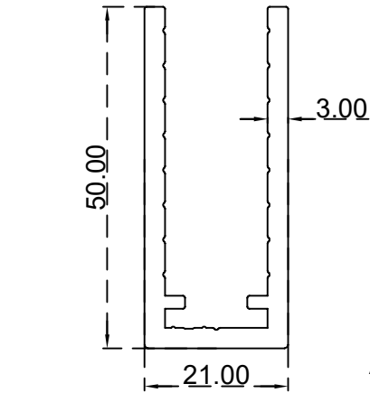
يو زجاج (21*50) ملم الرقم التسلسلي للصنف: AS00039 الوزن 0.960: (Kg/m)
