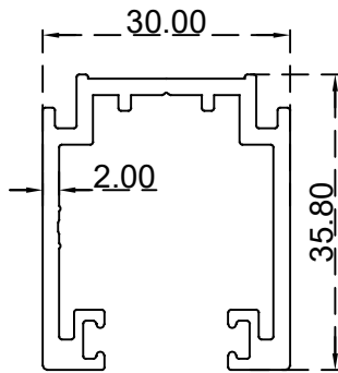
يو سقف الرقم التسلسلي للصنف: AS00049 الوزن 0.691: (Kg/m)
