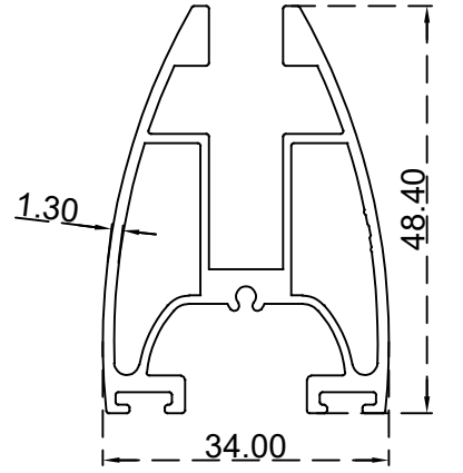
دفة تلسكوب الرقم التسلسلي للصنف: AS00063 الوزن 0.883:(Kg/m)
