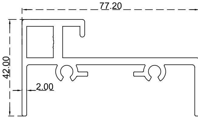
عليون تقطيع مكاتب الرقم التسلسلي للصنف: AS00073 الوزن 1.565:(Kg/m)
