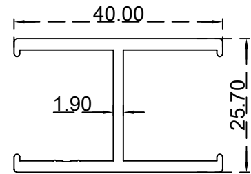
قاطع سنجل الرقم التسلسلي للصنف: AS00096 الوزن 0.602:(Kg/m)
