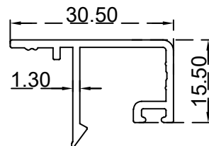
كلبس زجاج 15.5 ملم الرقم التسلسلي للصنف: AS00050 الوزن 0.287: (Kg/m)
