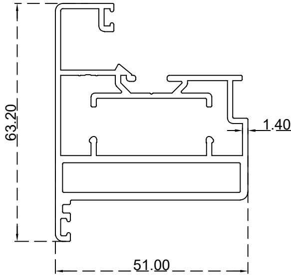
حلق باب الرقم التسلسلي للصنف: AS00052 الوزن 1.413:(Kg/m)
