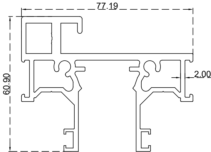
جنب تقطيع مكاتب الرقم التسلسلي للصنف: AS00074 الوزن 2.336:(Kg/m)
