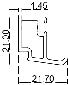
كلبس زجاج 8 ملم الرقم التسلسلي للصنف: AS00100 الوزن 0.280: (Kg/m)
