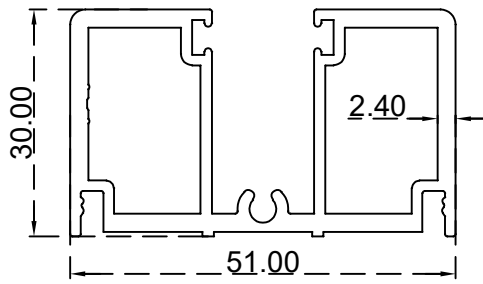
يو جانبي الرقم التسلسلي للصنف: AS00058 الوزن 1.130:(Kg/m)
