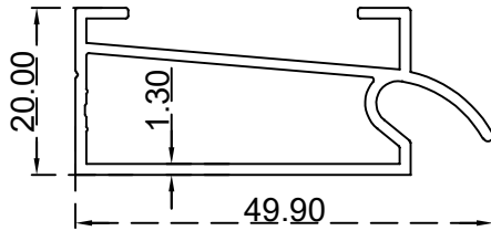
رداد ماء تلسكوب الرقم التسلسلي للصنف: AS00064 الوزن 0.485:(Kg/m)
