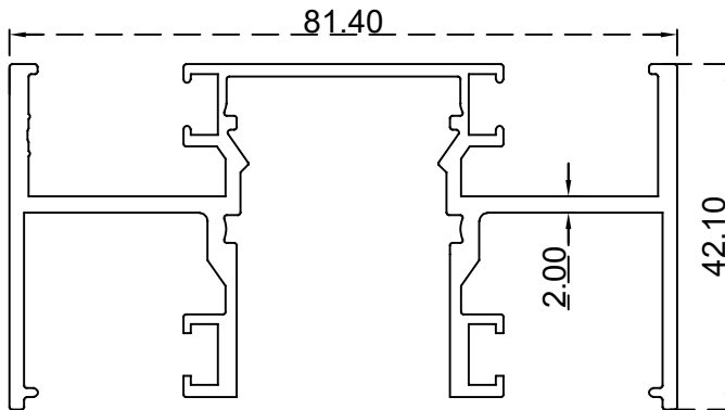
جنب تقطيع مكاتب الرقم التسلسلي للصنف: AS00074 الوزن 2.336:(Kg/m)
