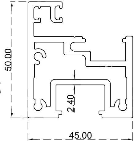
حلق الرقم التسلسلي للصنف: AS00041 الوزن 1.726: (Kg/m)
