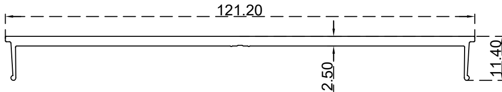
غطاء علبة كهرباء الرقم التسلسلي للصنف: AS00061 الوزن 0.863:(Kg/m)
