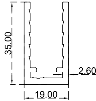
يو زجاج (19*35) ملم الرقم التسلسلي للصنف: AS00040 الوزن 0.611: (Kg/m)
